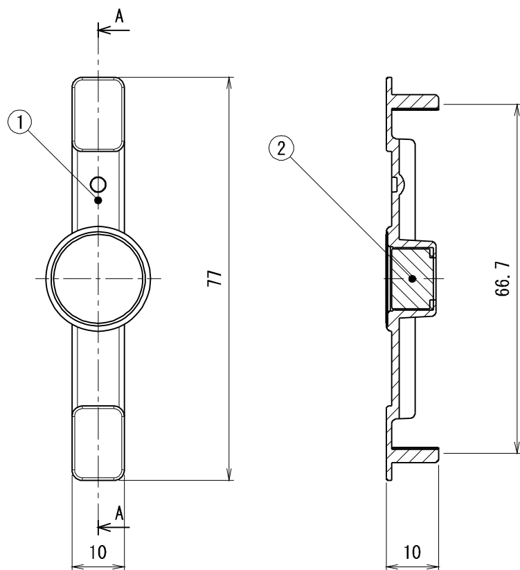
断面 A-A
